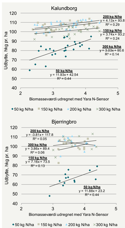
FIGUR 11. Udbyttet i forsøgene i Kalundborg og Bjerringbro ved 50, 150, 200 og 300 kg kvælstof pr. ha som funktion af biomasseværdien målt med Yara N-Sensor medio april før anden gødsning.
